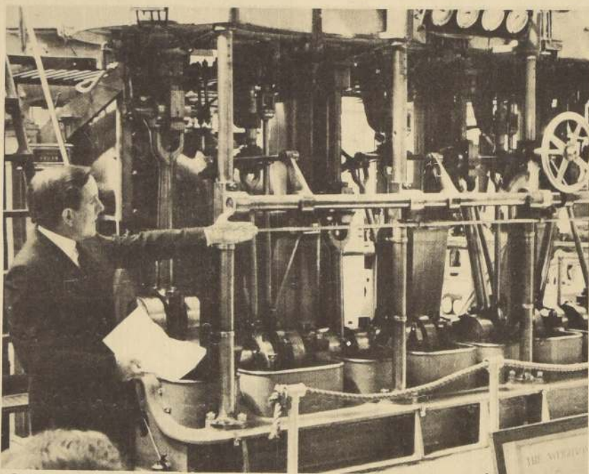
El motor Weighton, diseñado en 1894 por el profesor R. L. Weighton del King's College, ahora Universidad de Newcastle, en el noroeste de Inglaterra, diseñado especialmente para resolver los problemas de la máquina de vapor, ha sido cedido recientemente
