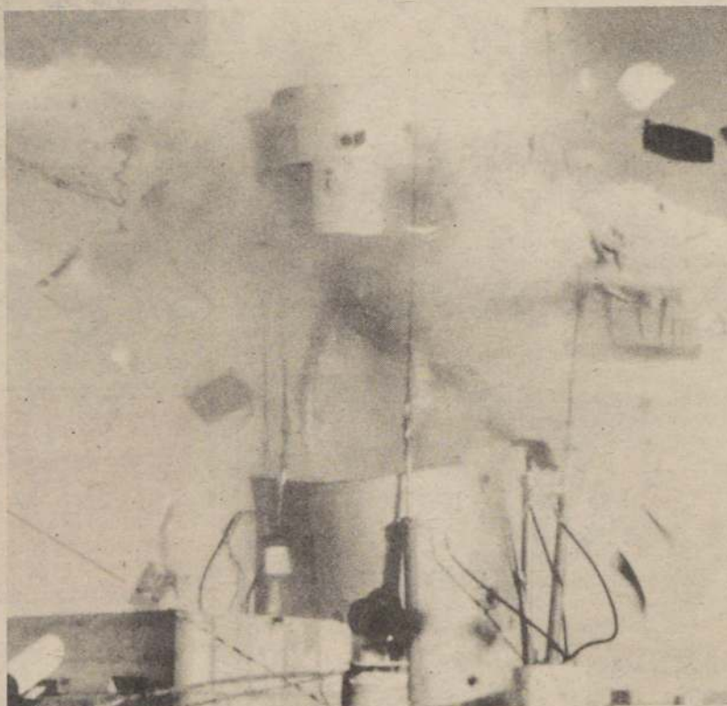
La segunda etapa de un cohete propulsor de misiles Titán I es destruida segundos después de ser irradiada con un rayo láser de alta energía en el Campo de Misiles White Sands en Nueva México. Esta primera prueba del poder mortífero del láser fue llevada a cabo como parte de la investigación relacionada con la Iniciativa de Defensa Estratégica de Estados Unidos. (USIS).
