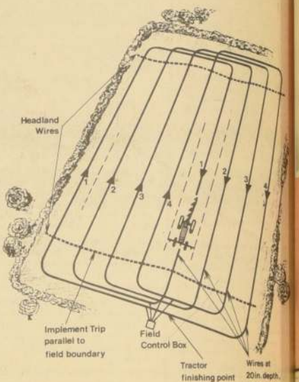
Colocación idónea de los alambres de dirección, que se entierran bajo el terreno para conducir al "Autotrack".
