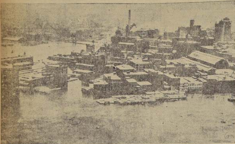
El barrio de la ciudad de Pittsburgh, conocido con el nombre de el Triángulo de Oro, transformado en una isla, a raíz de las inundaciones recientes
