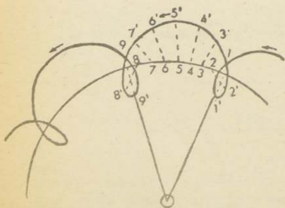
Fig. 82— Representación de las órbitas epícicloides de los planetas
