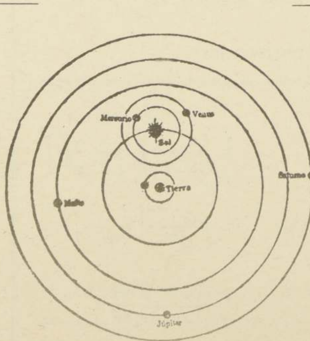
Fig. 84— Representación del sistema solar, según Tycho-Brahe
