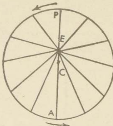
Fig. 83— Representación de la excéntrica, según las ideas de Hiparco y de Ptolomeo
