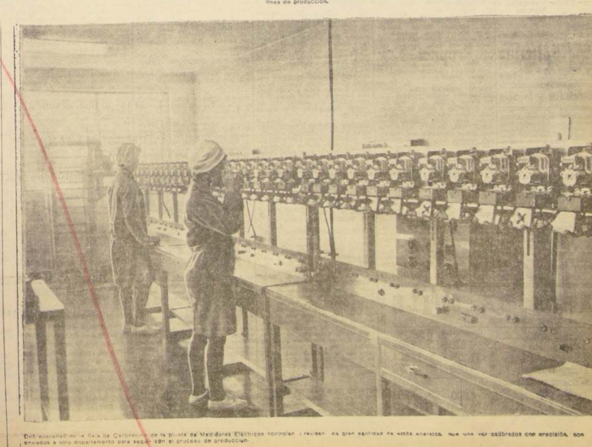
Del laboratorio de la Sala de Calibración de la planta de Medidores Eléctricos controlan y revisan las gran cantidad de estos aparatos, que una vez calibrados con exactitud, son enviados a otro departamento para seguir con el proceso de producción.
