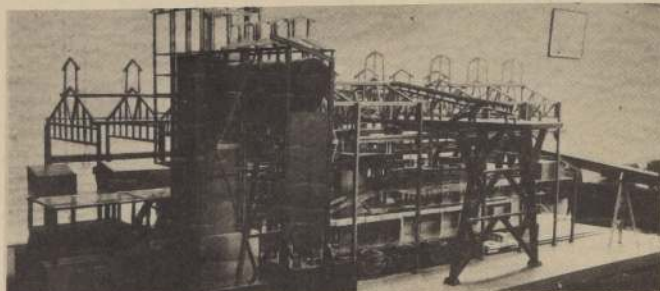
CON UN NUEVO HORNO REVERBERO contará, a partir del mes de mayo, la Fundación de Calesones del Mineral "El Teniente". La nueva obra permitirá aumentar la actual producción de cobre fino en 200 toneladas, con equivalencia de US$ 200 mil por día. Vale decir, que la Fundación quedará en condiciones de entregar al país unas 900 toneladas de cobre al día. El nuevo horno fue ejecutado y diseñado enteramente por trabajadores chilenos y, por primera vez, no ha sido necesario pagar a otros países por licencias o patentes extranjeras. También se han aprovechado todos los recursos nacionales con respecto a materiales y equipos. Ello permitió mantener el gasto de divisas en apenas un 10% de la inversión total, que alcanza a 120 millones de pesos. El desafío del moderno horno reverbero, que concentra las técnicas más avanzadas sobre fundición, comenzó en el mes de enero del año pasado y en él participaron aproximadamente 300 trabajadores. EN LA FOTO un modelo a escala del horno con que contará la Fundación de Calesones.
