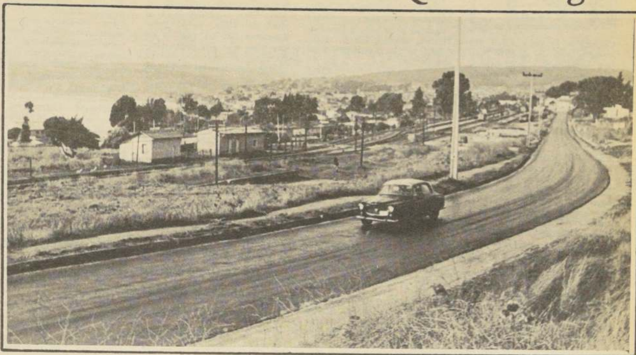
EL NUEVO pavimento asfáltico en el camino de San Antonio a Algarrobo. Obsérvese que se ha eliminado el lomo excesivo de la calzada, lo cual evitará el desnivel y el peligro de volcamiento de los vehículos.
