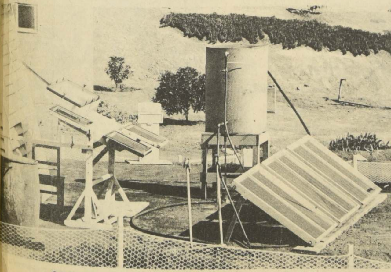
CALENTADOR SOLAR, construido en la Universidad del Norte.
