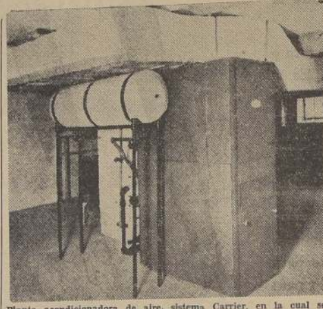
Planta acondicionadora de aire, sistema Carrier, en la cual se verifica el proceso completo de climatización.
