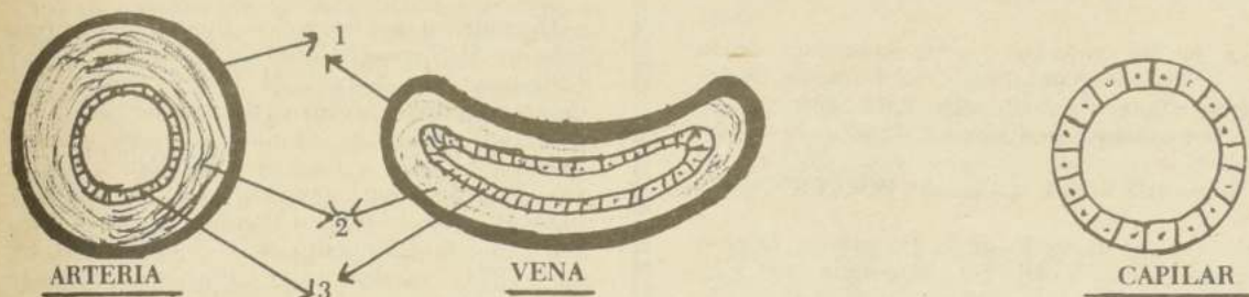
Esquema comparativo de la estructura de los vasos sanguíneos
