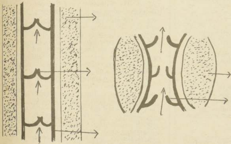
Esquema que explica la circulación venosa:
