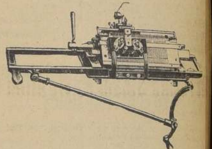
Primitiva máquina de tejer "Clas"
