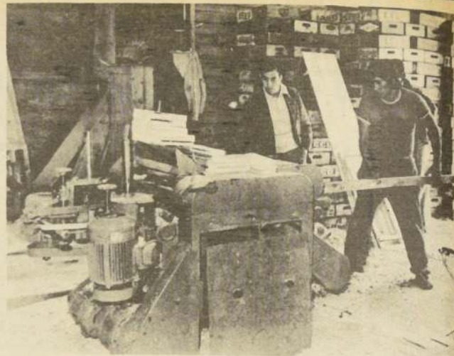
LA CEPILLADORA eléctrica adquirida recientemente constituye una de las máquinas claves en el moderno taller de carpintería de la Cárcel de Valparaíso.
