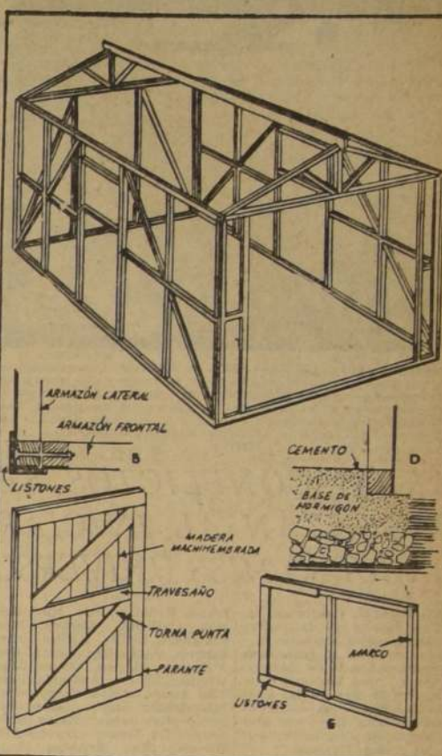
Garage desarmable de 4.50 metros por 3 metros.
