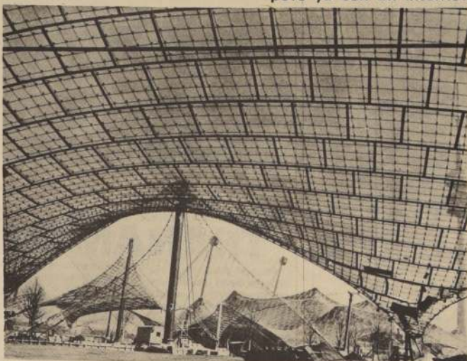
El tejado de las pistas, cuando aún estaba en construcción. Es el mayor del mundo.
