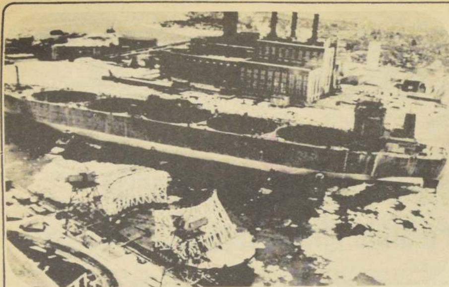
BARCO CISTERNA DE GAS, (Quincy), Massachusetts. Este es el primero de los 12 enormes barcos-cisternas para distribución del gas natural. Se ve cuando abandona los astilleros por sus propios medios. La nave será sometida a pruebas antes de que se le coloquen esferas para cubrir los tanques de gas. (Foto AP).
