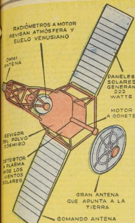
El esquema del famoso Mariner II, que en estos momentos va en viaje al planeta Venus.
