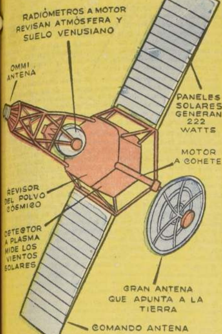
El esquema del famoso Mariner II, que en estos momentos va en viaje al planeta Venus.
