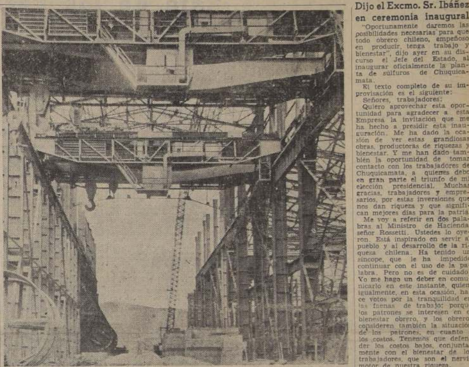
PLANTA DE SULFUROS DE CHUQUICAMATA INAUGURO S. E. AYER.— Con un costo de 120 millones de dólares, la Chilex Exploration Co. levantó en Chuquicamata una nueva planta de sulfuros para el tratamiento del cobre, con un menor costo, mayor rendimiento y mejor recuperación. A las ceremonias inaugurales asistieron el Jefe del Estado y los Ministros de Hacienda, Juan Rossetti; de Obras Públicas, don Orlando Latorre, y del Trabajo, don Leandro Moreno. El Ministro Rossetti, hablando a nombre del Gobierno, expresó ayer su "complicencia" por esta obra magnífica, que el empuje y la técnica norteamericana, asociada al esfuerzo de los trabajadores de Chile, hicieron una realidad. En el grabado vemos un aspecto de los Molinos de esta nueva planta.
