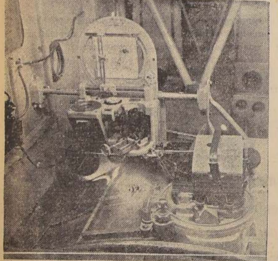
La cámara métrica fotográfica automática y el "Quo Vadis" montado en la cabina del avión destinado al trabajo aéreo de levantamiento.
