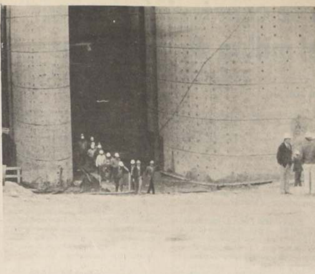
Los túneles de desviación del río Maule, paso previo para la construcción del embalse Colbún, en el proyecto hidroeléctrico Colbún-Machicura, están llegando a su término. En el grabado, el Intendente Sergio Pérez recorre el túnel, el más largo de este tipo existente en el país.
