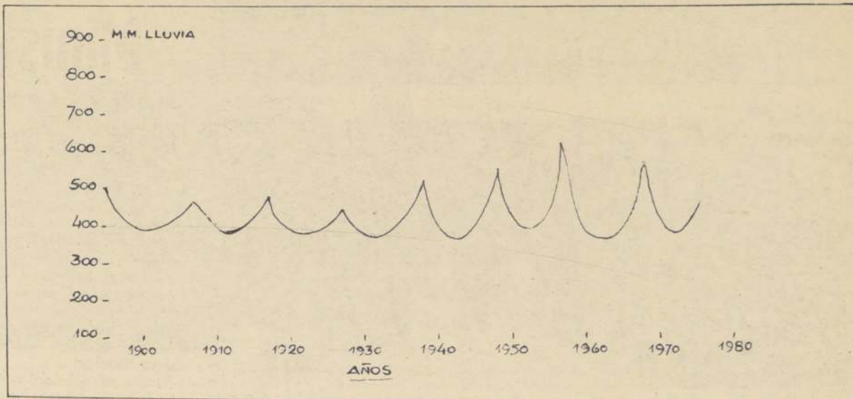
El gráfico muestra la periodicidad de épocas lluviosas y secas, señaladas en milímetros de agua caída (verticales) según los años (horizontales), desde principios de siglo.
