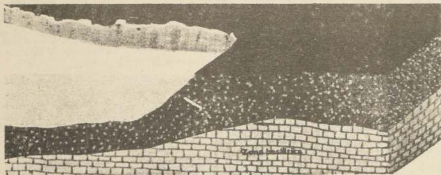
Capas que constituyen la litosfera
