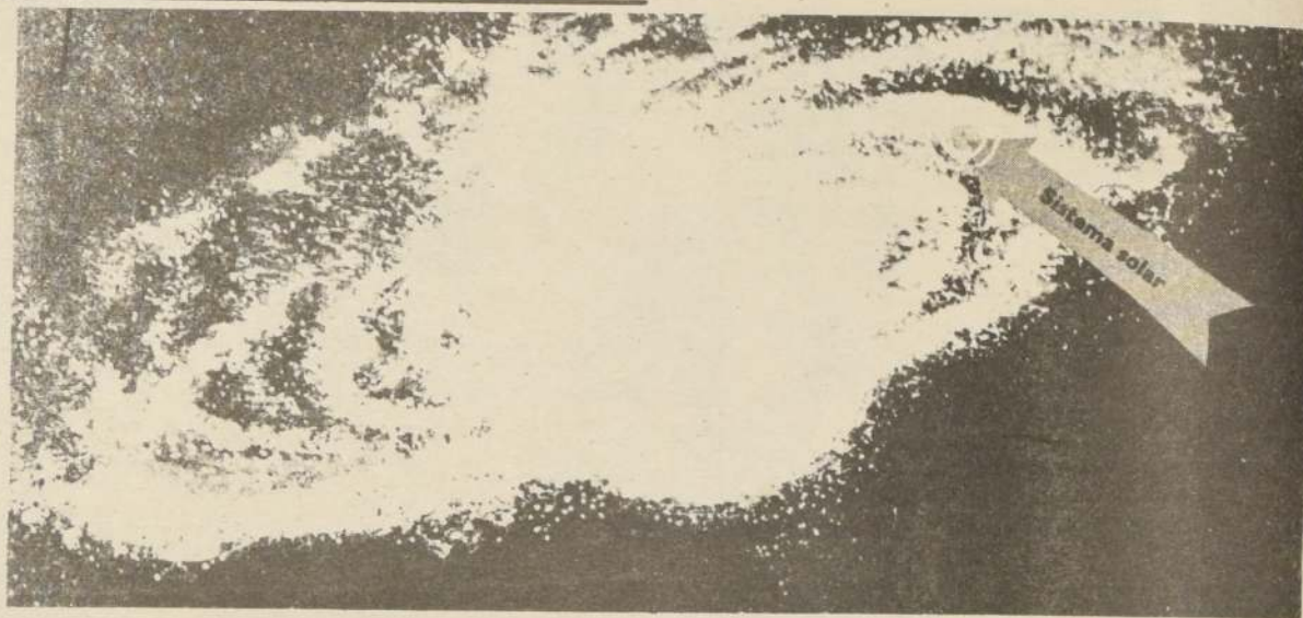
Situación del Sistema Solar en la Vía Láctea.
