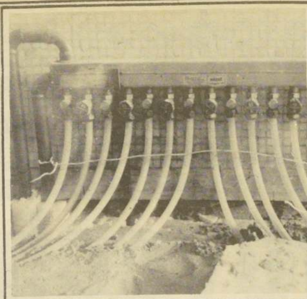
SISTEMA de distribución del agua caliente en el hospital de Combarbalá, primero en Chile que contará con calefactores a energía solar.
