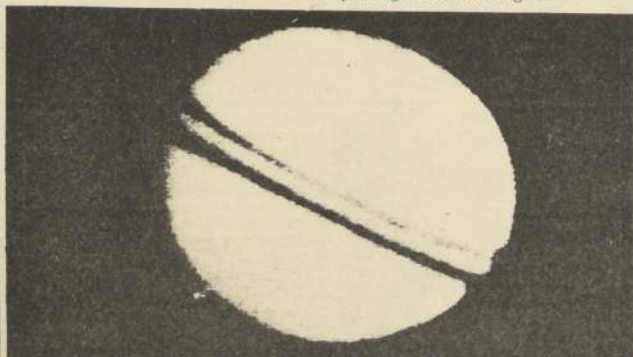
Imagen lograda por el Pioneer 11, a la distancia de 3.425 millas de Saturno. El contraste se logró por computador, utilizando un procedimiento que sacrifica la prolongación de los anillos en la atmósfera.
