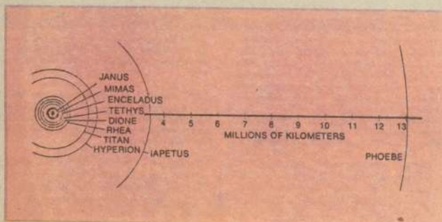
Órbitas de las lunas de Saturno. Las ocho más cercanas al planeta son casi circulares y no se desvían más de 2 grados del plano del Ecuador. La órbita de Iapetus tiene una inclinación de 15 grados. Phoebe gira en órbita inclinada de 150 grados, muy excéntrica y puede ser un objeto captado. Los anillos están muy próximos a Saturno y no alcanzan a figurar, por la escala del dibujo
