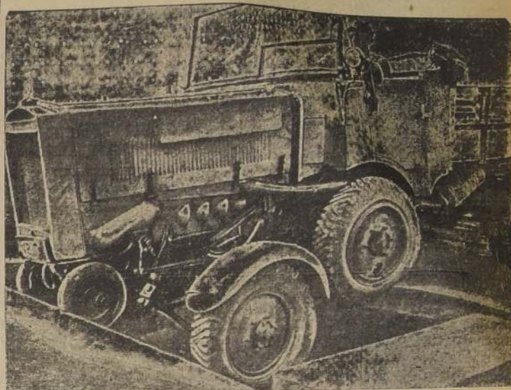
El camión que aparece en el grabado fue construido por la Fábrica Mercedes Benz y puede salvar cualquier obstáculo del camino gracias a la novedosa disposición de las ruedas. Se trata de un vehículo provisto de ocho ruedas motrices con suspensión individual con movimientos perfectamente calculados para permitir el paso de un foso como el que muestra el grabado o cualquier otro accidente
