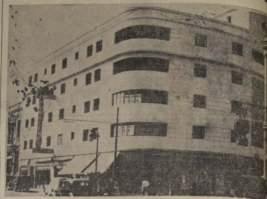
En Alameda Bernardo O'Higgins esquina de San Alfonso, se ha terminado la construcción de la obra un magnífico edificio para hotel. Arquitecto: don Luis Vergara Larraín; Cálculos de Resistencia, don Guillermo Camus. Contratista general, D. Miguel Sancho B.
