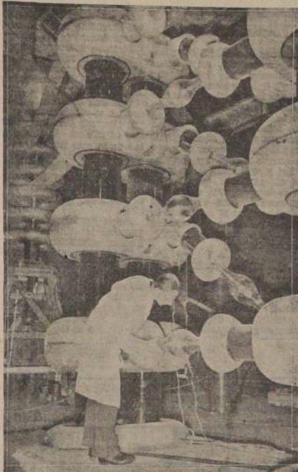
El enorme generador de alta tensión para producir 1.200.000 voltios.
