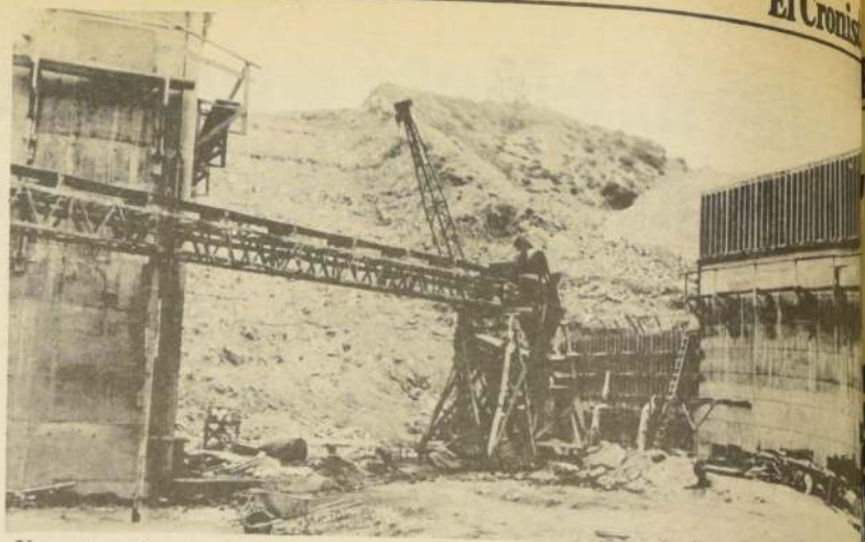
Un aspecto de la construcción del "rápido de descarga" del embalse "Aromos" sobre el estero Limache.
