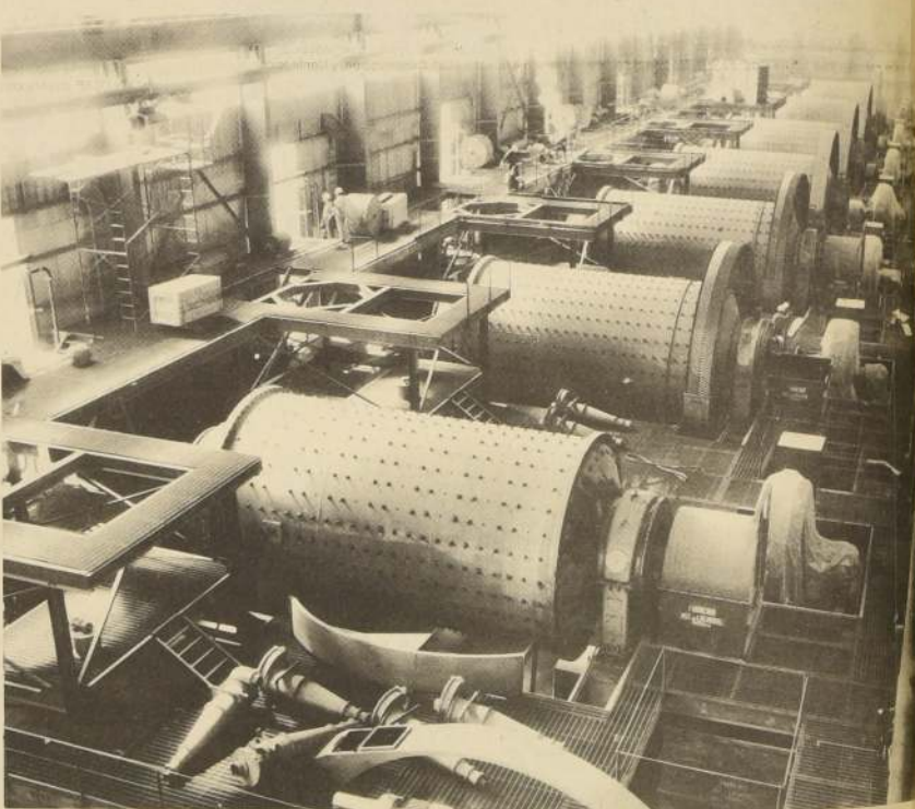
LOS NUEVOS MOLINOS DEL CONCENTRADOR "COLÓN" DE LA SOCIEDAD MINERA "EL TENIENTE"
