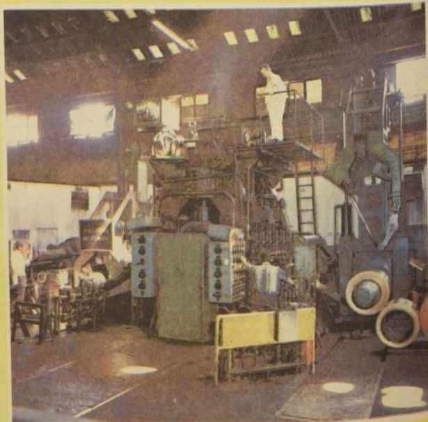
NUEVAS instalaciones de trefiladoras de tubos de cobre en rollos para conducción de fluidos líquidos y gaseosos y ductos eléctricos, en instalaciones urbanas domiciliarias e industrias varias.
