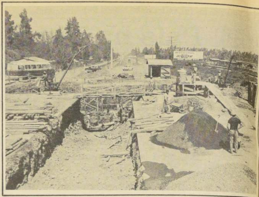
PUENTE de Santa Marta facilitará el acceso a San Antonio.
