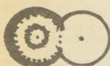
Molécula di-atómica de compuesto binario
