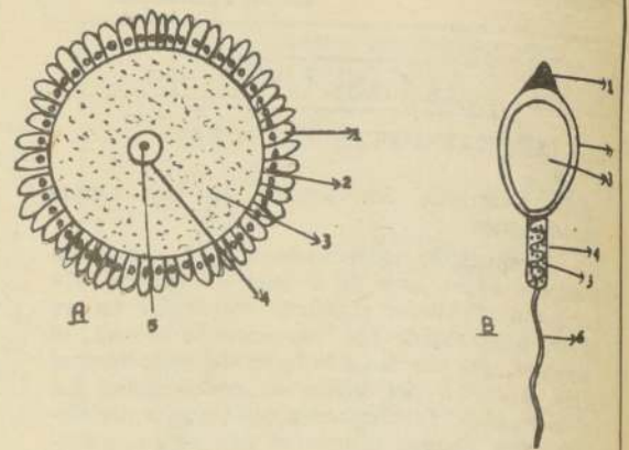
Esquema comparativo de los gametos femeninos (óvulo) y masculino (espermio)
