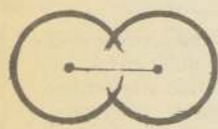
Molécula di-atómica de elemento
