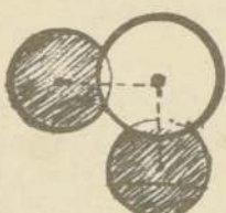
Molécula tri-atómica de compuesto
