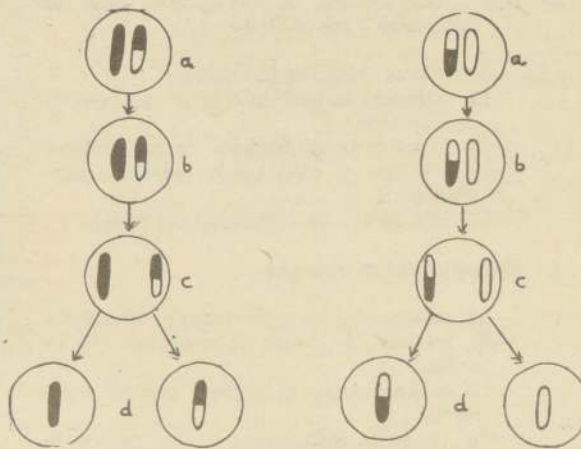
Representación de la segunda división meiótica
