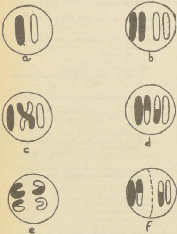
Representación de la primera división meiótica
