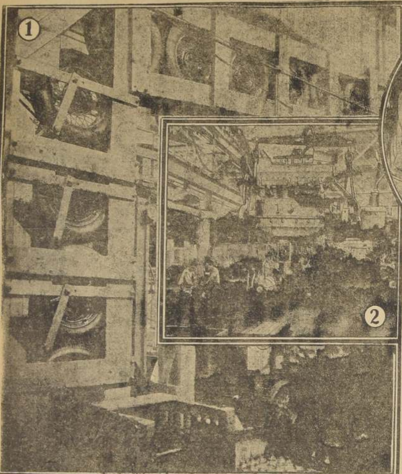
1. RUEDA TRANSMISORA QUE CONDUCE A LAS "RUEDAS" HASTA LA LINEA Y AL PUNTO NECESARIO. — 2. VISTA DE LA LINEA DE AGRUPAMIENTO DEL CHASSIS, EN UNA FABRICA DE DETROIT. LA GRUA DE LA PARTE SUPERIOR DEJA CAER EL ARMAZON EN EL SITIO NECESARIO. — 3. COLOCANDO LOS RESORTES Y EJES, MIENTRAS EL CHASSIS ESTA INVERTIDO. NOTESE LAS TENAZAS AUTOMATICAS QUE PENDEN DEL TROLLEY. — 4. CADA MAQUINA ES SUJETA A UNA PRUEBA ANTES DE SER COLOCADA EN EL CHASSIS.
