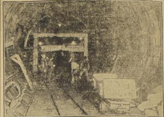
Cabecera de una de las secciones del túnel de la Ford ilustrando la maquinaria usada para horadar bajo tierra. Al frente se ven a las planchas de concreto que se usaron para forrar el túnel. Este tiene un diámetro interior de 15 pies.
