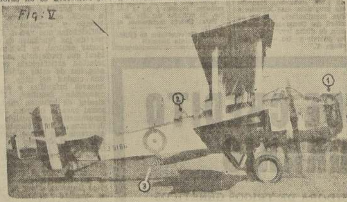
Bombardero diurno pesado, inglés, Boulton Paul "Overstrand", con dos motores 2450 P. S. Bristol "Pegasus". El avión posee tres posiciones de ametralladoras, de las cuales la una se encuentra en una torre giratoria blindada en la proa del avión (1), una posición abierta es situada en el centro del avión; (2), mientras un tercer tirador maneja su ametralladora cuerpo a tierra en el suelo del aparato (3).
