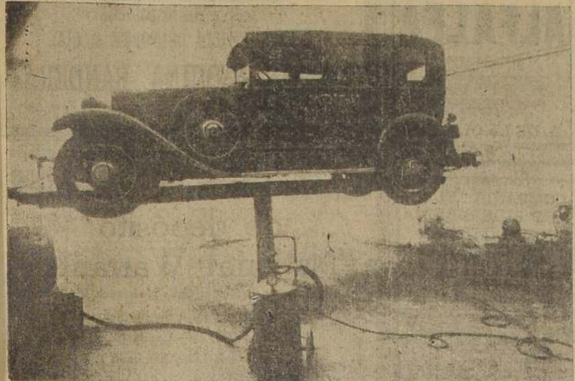
Departamento de engrase con su rampa giratoria.
