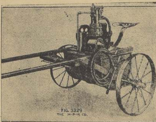
Moto-Bomba Pulverizadora Deming
