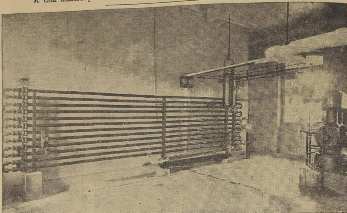
La máquina compresora y el condensador de frío
