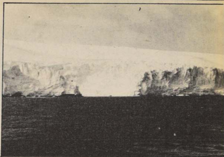
Lo escarpado de las costas antárticas presenta serias dificultades a los científicos que realizan el crucero geológico del INACH.
