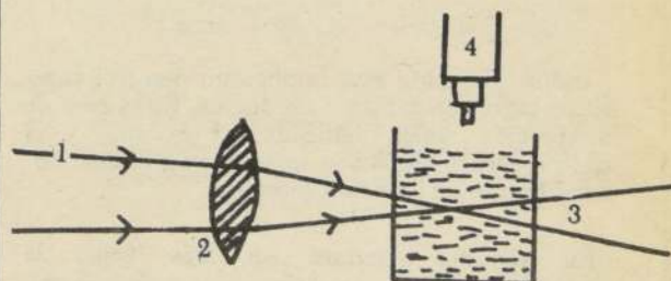
Esquema del ultramicroscopio en que se demuestra el efecto Tyndall
