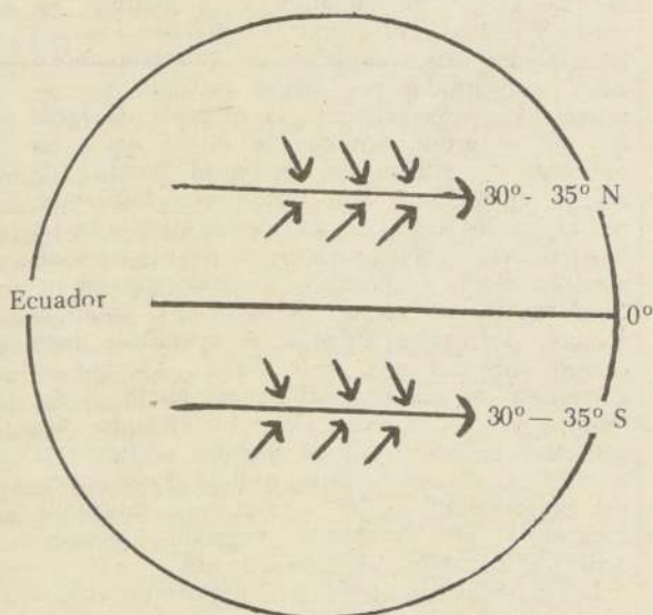
Representación de Corrientes de aire JET STREAM
