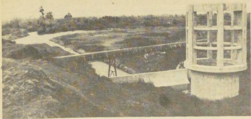
En la fotografía se ven las obras de toma de agua en el embalse de Convento Viejo. Para proseguir los trabajos, el Ministerio de Obras Públicas llamará a propuestas durante el curso del presente mes.
