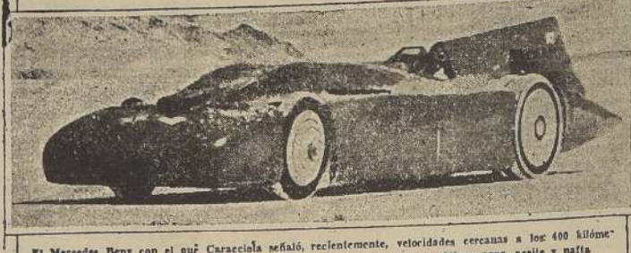
El Mercedes-Benz con el que Caracciola señaló, recientemente, velocidades cercanas a los 400 kilómetros. Tiene un motor de 600 HP, y pesa 750 kilogramos, sin neumáticos, agua, aceite y nafta.
