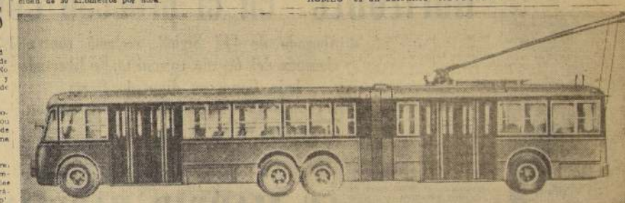
El grabado representa un autobús Alfa Romeo "140 AFS/4", con capacidad para 160 personas. Tiene un largo de 17,5 metros y un radio de viraje de 12 metros. Su velocidad aproximada es de 50 kilómetros por hora y su potencia es de 200 HP. Está dotado de cuatro sistemas de frenos: neumático de pedal, mecánico a mano en las ruedas motrices, freno eléctrico y freno neumático de socorro. La Alfa fabrica, además, un modelo no articulado, con capacidad para 105 pasajeros.
