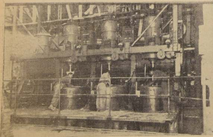
Otro grupo de maquinarias para la elaboración del azúcar en la Compañía Refinería de Azúcar de Santiago
