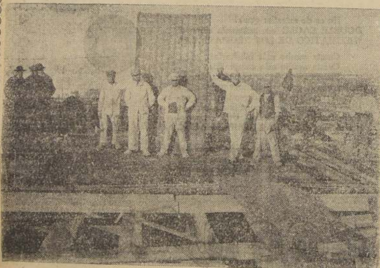
El Solomite empleado como material de cofraje, bajo pisos y tabiquería en el Gran Hotel de Ibbarta (1928 - 1929). Este Solomite es de paja común (paneles de 3.50 por 1.50 m.). La colocación costó 50 céntimos franceses por metro cuadrado.
