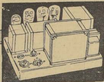
Nueva amplificación Victor equilibrada. Emplea dos nuevos tipos de radiotrones RCA No. UX245. Produce mayor energía. Funcionamiento económico.
