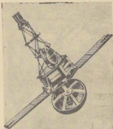
El Mariner II, astronave norteamericana que el 14 de diciembre último alcanzó su punto de mayor proximidad con el planeta Venus.
