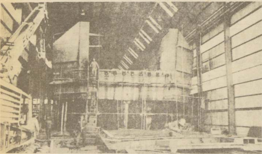
EL 20 DE DICIEMBRE los Astilleros ASENNAV de Valdivia entregarán terminado a Transmarchilay el transbordador "El Colono", que unirá Quellón con Puerto Chacabuco. La foto muestra la primera etapa de construcción de esta embarcación.
