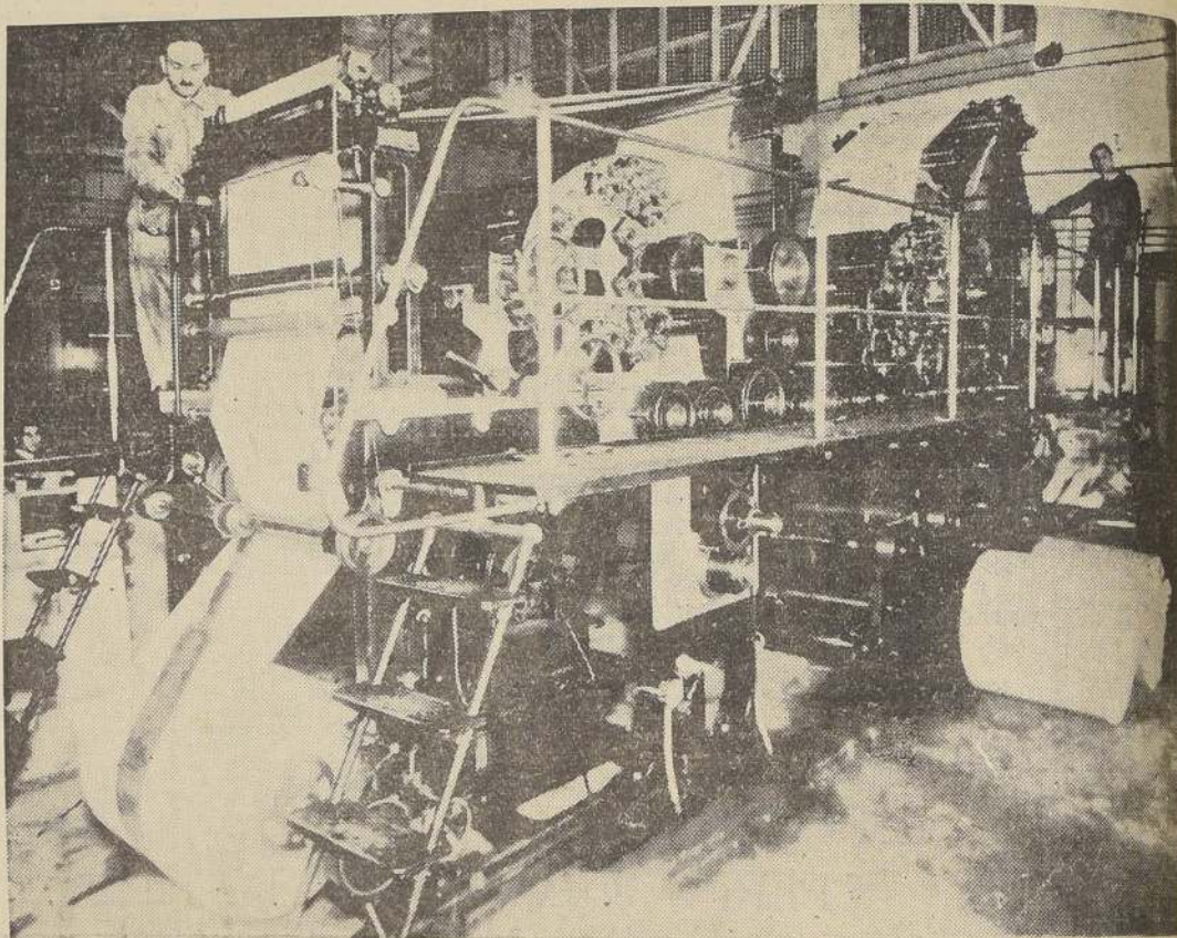
Maschinenfabrik Augsburg Nürnberg. Prensa rotativa M. A. N. para impresiones de alta calidad, de propiedad de la Editorial Ercilla que funciona en sus talleres y que es la primera prensa rotativa para la impresión de libros en Hispano América.
