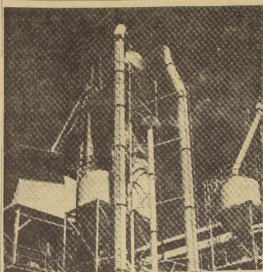
PLANTA DE FERTILIZANTES.— La industria de Israel, aprovechando el denodado esfuerzo de sus técnicos y obreros, ha logrado levantar los múltiples aspectos fabriles a extremos que, hace seis años, eran imposibles de prever. El grabado muestra parte de la planta de fertilizantes y productos químicos, existente en la bahía de Haifa.
