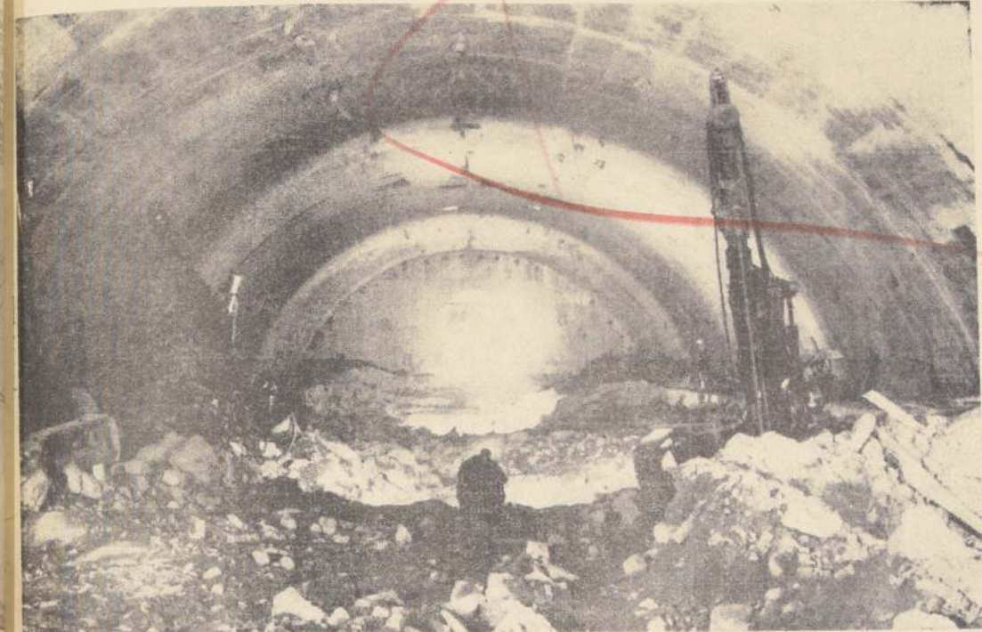
El Toro, una vez en funcionamiento, será el segundo gran aprovechamiento hidroeléctrico de los caudales del lago Laja, después de la central Abanico. Como obra de ingeniería también constituirá una realización excepcional, ya que será enteramente subterránea, incluso su casa de máquinas. Captará el agua del Lago a 80 metros de profundidad y un túnel de 9 kilómetros —que cruzará la cordillera de Polcura— la conducirá hasta las tuberías de presión, de casi un kilómetro y medio de longitud, a través de las cuales llegará hasta las turbinas de la casa de máquinas, con una altura de caída de 610 metros.
