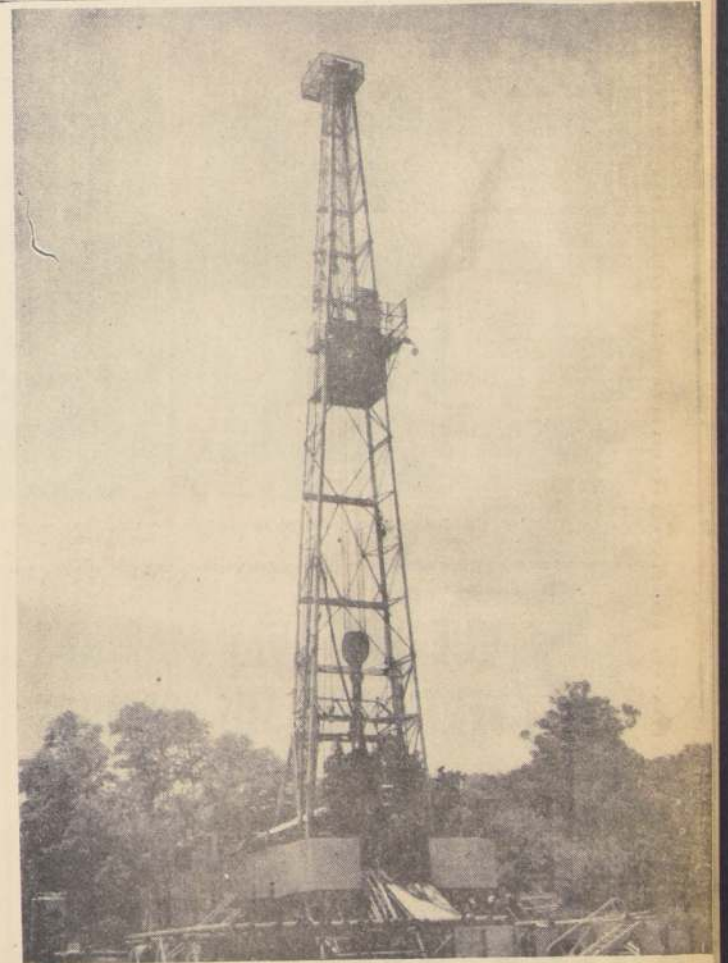
Una pesada torre de perforación con todo su equipo anexo fue trasladada hasta Arauco por la ENAP, a fin de realizar perforaciones. Cerca de Lebu se han horadado diez pozos, el número uno resultó estéril y el dos arrojó gas natural. Ahora, como se puede apreciar en el grabado se está trabajando un tercer pozo.
