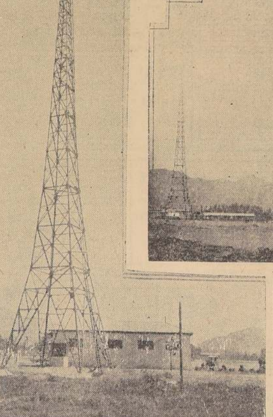
Una de las torres metálicas de la radio-estación de Copiapó.
