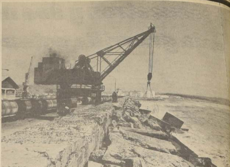
Un aspecto de las gigantescas obras que se están ejecutando en el puerto de San Antonio, en la construcción del nuevo sitio de atraque.
