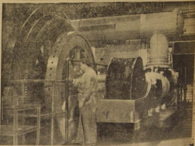
PODEROSAS MAQUINARIAS. —En el interior de la mina se han instalado maquinarias de gran volumen. La subestación, a 500 metros de profundidad horizontal y 500 de profundidad vertical, proporciona abundante iluminación y energía para mover todo el sistema interior de la mina y las instalaciones de aire acondicionado.
