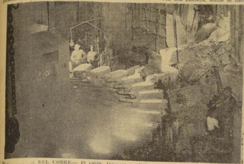
LOS MOLD'S DEL COBRE. —El cobre, fundido a alta temperatura, cae en estado líquido a los mold's de los lingotes, desde donde es llevado, automáticamente, a la sección "Enfriamiento".
